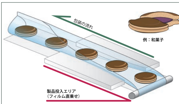
SP153Ron（直乗せ）の搬送方式（イメージ）
