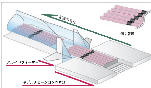
SP153Rの搬送方式（イメージ）
